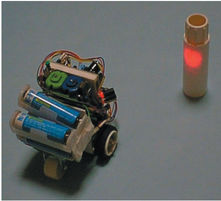
写真F スラローム走行ロボット(第6・3章)
