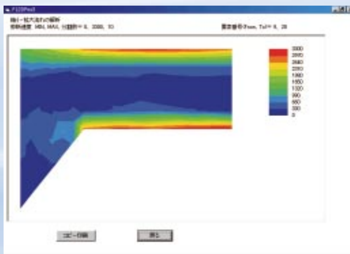
図8.42 縮小・拡大流れの縮小部の等高線図 (剪断速度, カラーフィル有り) 本文224ページ
