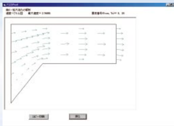
図8.41 縮小・拡大流れの縮小部の 速度ベクトル図。 本文224ページ
