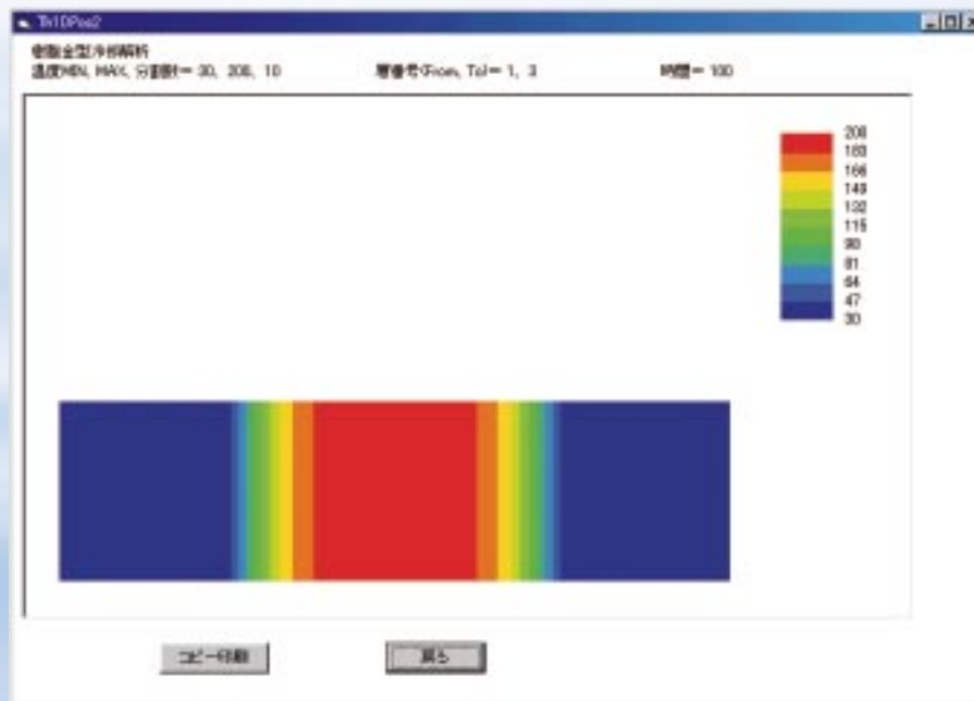
図6.27 樹脂金型冷却の等温線図 (カラーフィル有り). 本文149ページ
