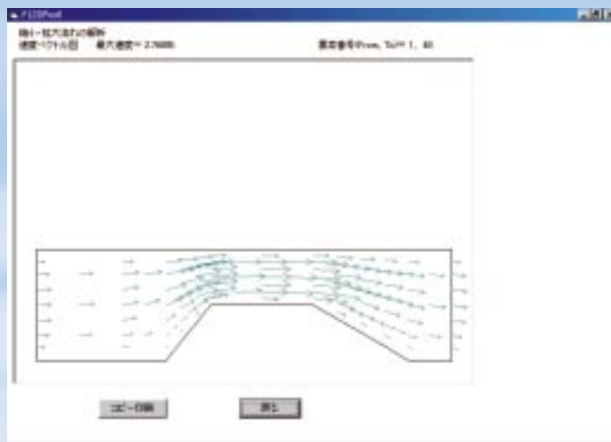
図8.40 縮小・拡大流れの 速度ベクトル図。 本文224ページ
