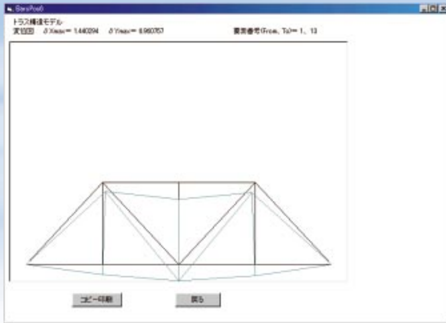
図7.25 変位図の作画画面．本文176ページ
