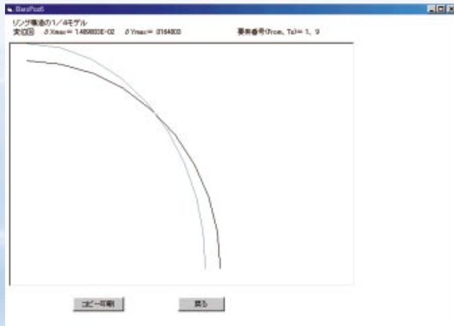
図7.27 リング構造の1/4モデルの変位図．本文176ページ
