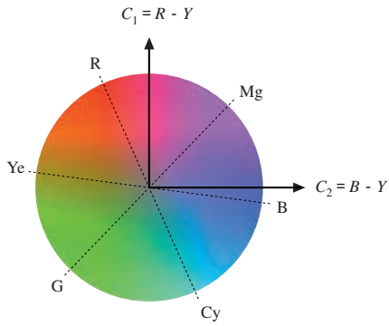
図6.7 Y = 127 のときのYCC色平面
