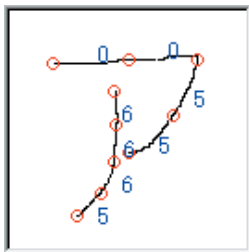
図5.10 方向コード列の実行例
