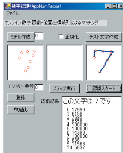
図5.17 プロジェクト実行画面（認識結果）
