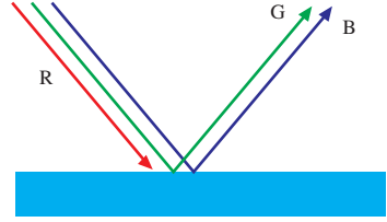
図6.3 インクによる発色 (シアン)
