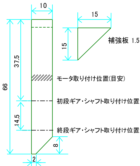
モータ・ギア・マウント 1.5mm バルサ
