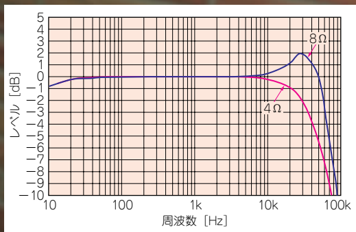
【周波数特性 (実測値)】
