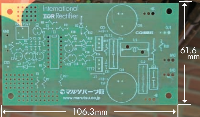
D級アンプ基板TR0803Dの 部品実装イメージ (部品は付録に含まれていません)
