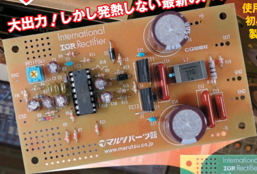
D級アンプ基板TR0803Dの 部品実装イメージ (部品は付録に含まれていません)
