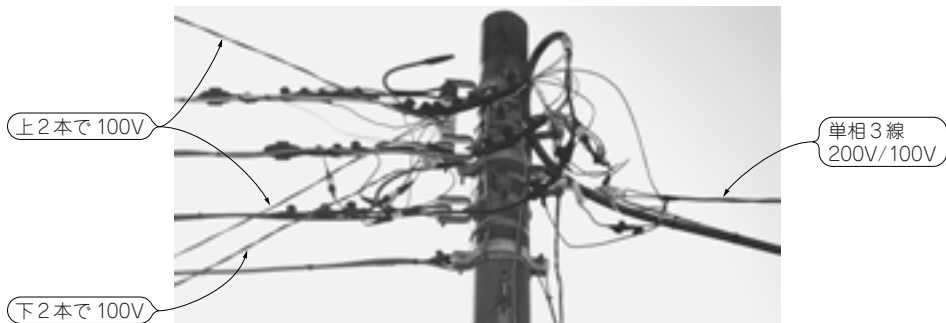
单相3線の電線から各家庭への100Vを引き出しているようす
