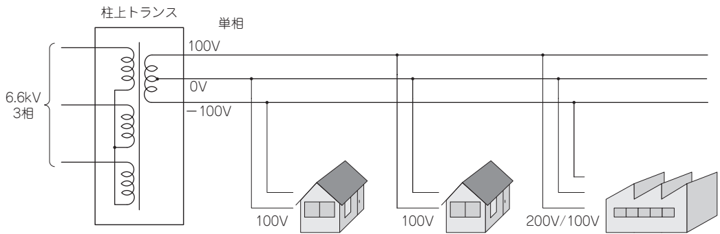
図6-2-3 200V/100Vの配電線の様子
