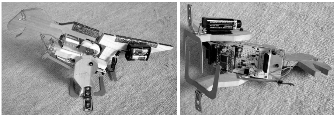
写真28 3664搭載の“恐竜ロボット”
