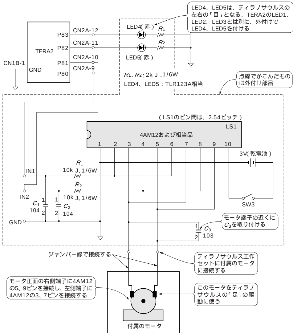
図31 ティラノサウルス制御回路
