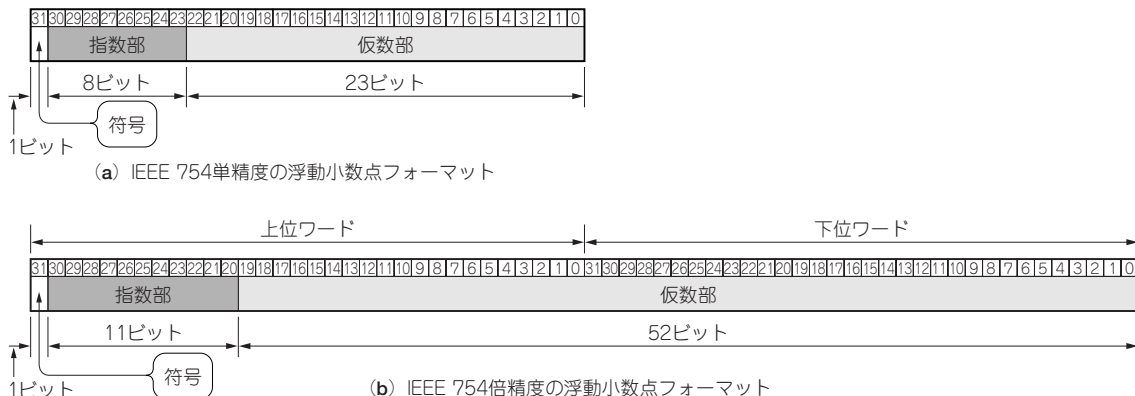
図6-4 浮動小数点形式
