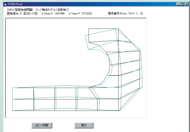
図 10.30 変位モード図の作画画面( フック , 比例 減衰でない MCK 型 ). 本文 188 ページ
