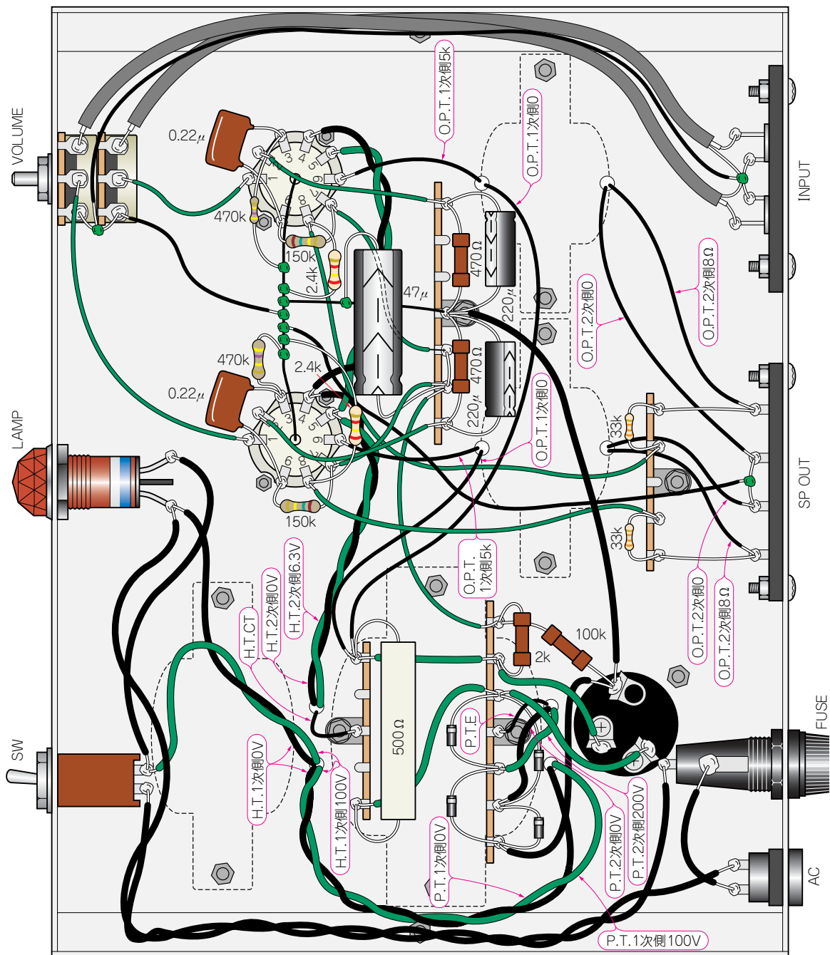
図1.3 6BM8 シングル・ステレオ・アンプの実体配線図
