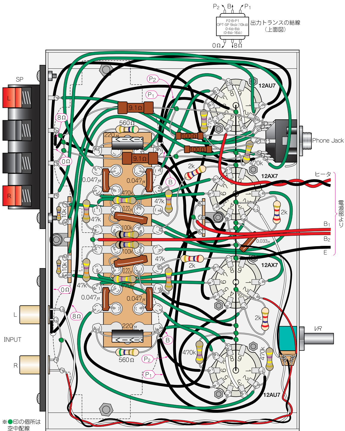
(b) 信号部
