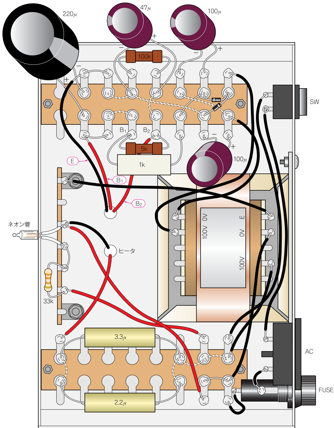
(a) 電源部
