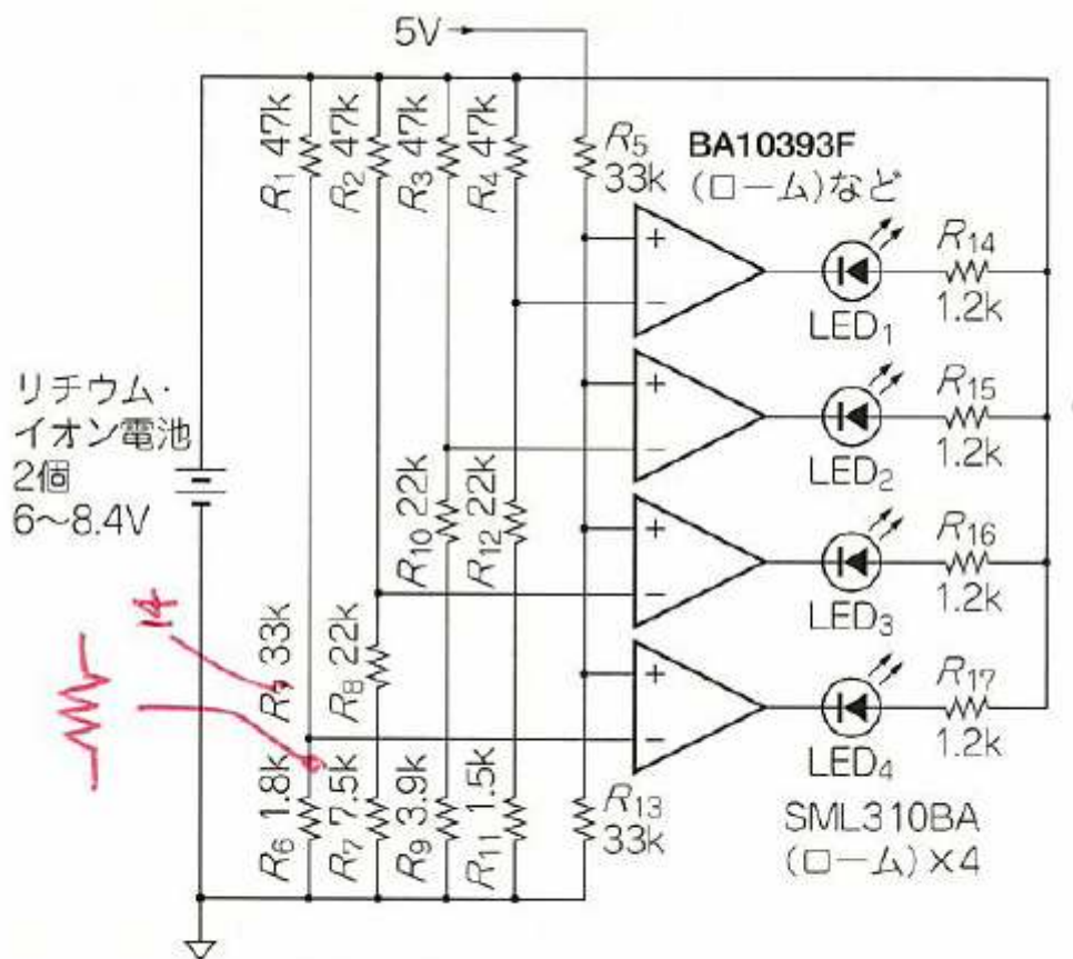
図 5-2 リチウム・イオン電池の残量表示回路
