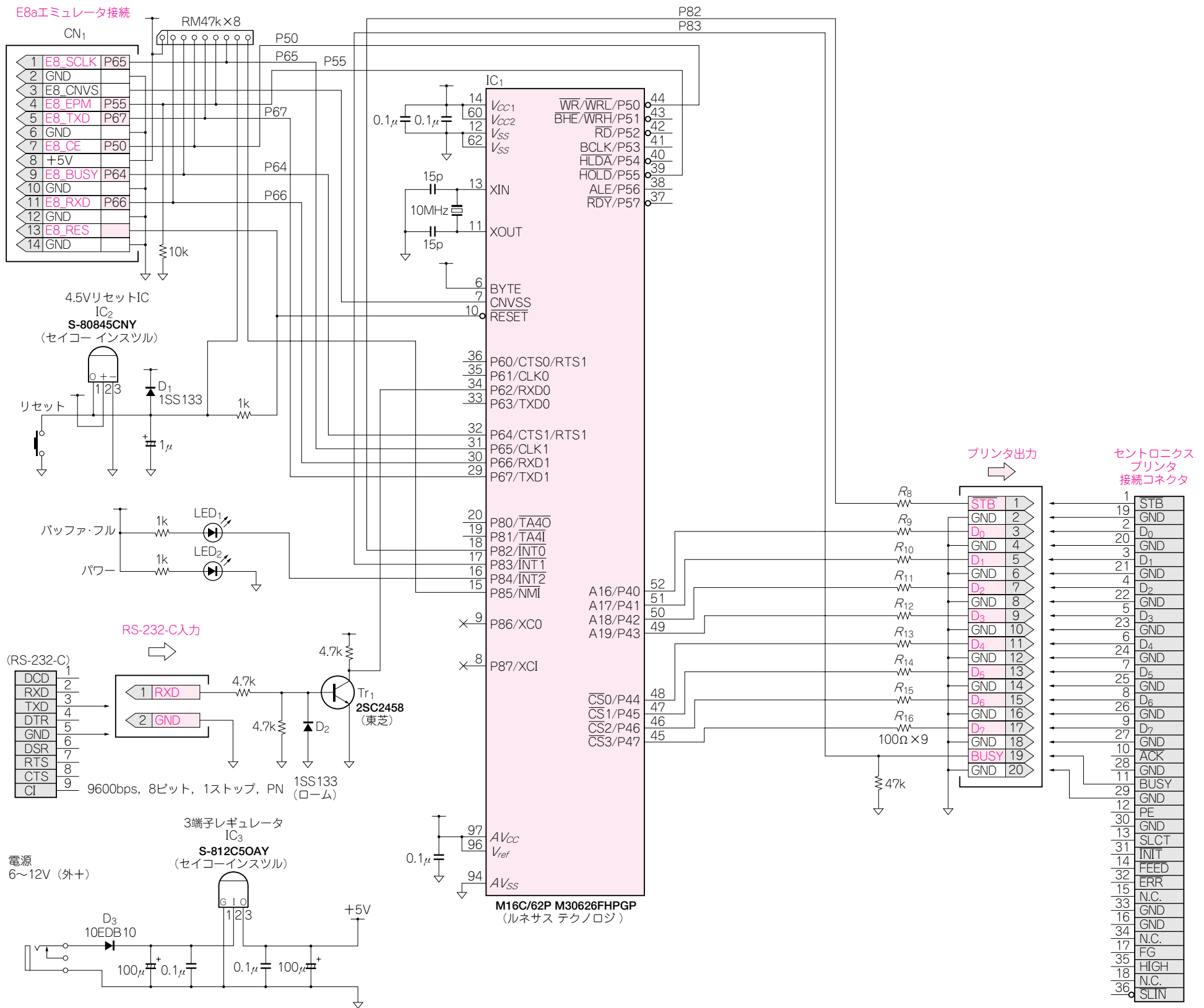
図11-1 M16C/62Pを使ったシリアル→パラレル変換回路
