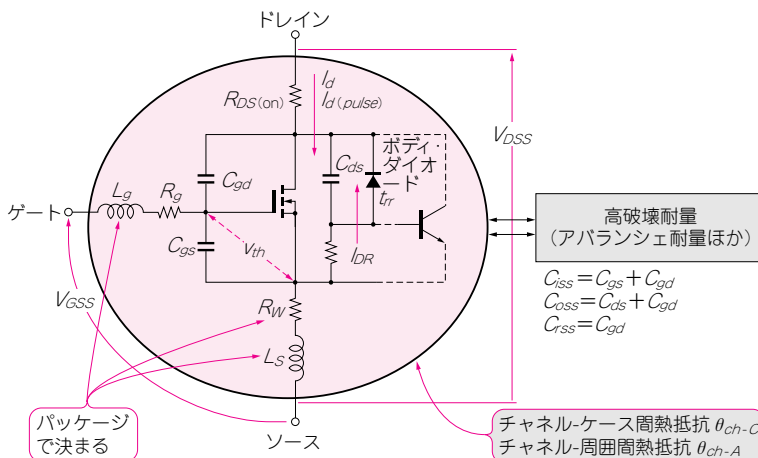
図3-1 パワー MOSFET の等価回路とキー・パラメータ
