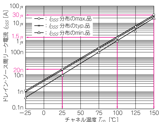
図3-2 ドレイン・ソース間リーク電流 I_{DSS} -チャネル温度 T_{ch} 温度依存性 (HAT2165H/LFPAK, V_{DSS} = 30 \text{ V} , R_{DS(on)} = 2.5 \text{ m}\Omega )
