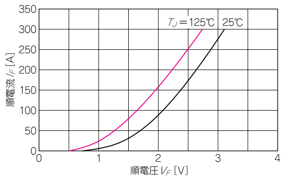
図5-2 FWD部の出力特性
