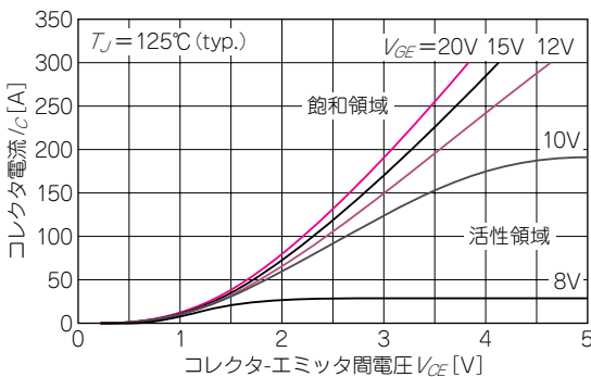
図5-1 IGBT部の出力特性
